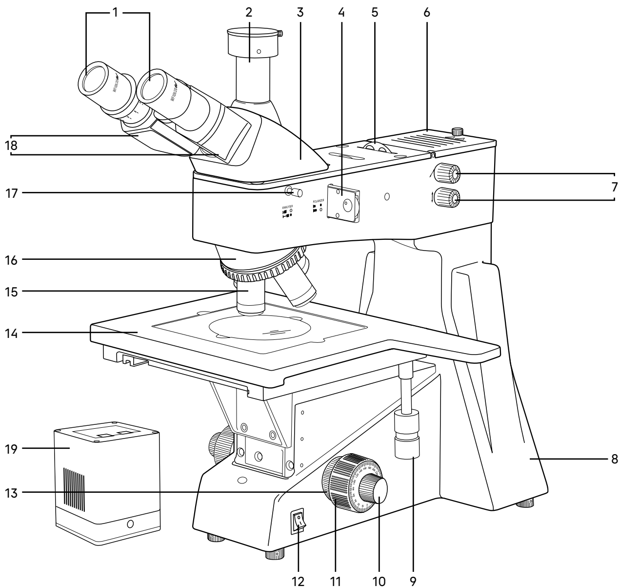
Рис. 1. Микроскоп MAGUS Metal D650 BD. Вид справа
