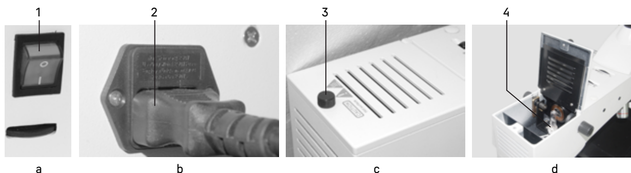
Рис. 18. Замена лампы
