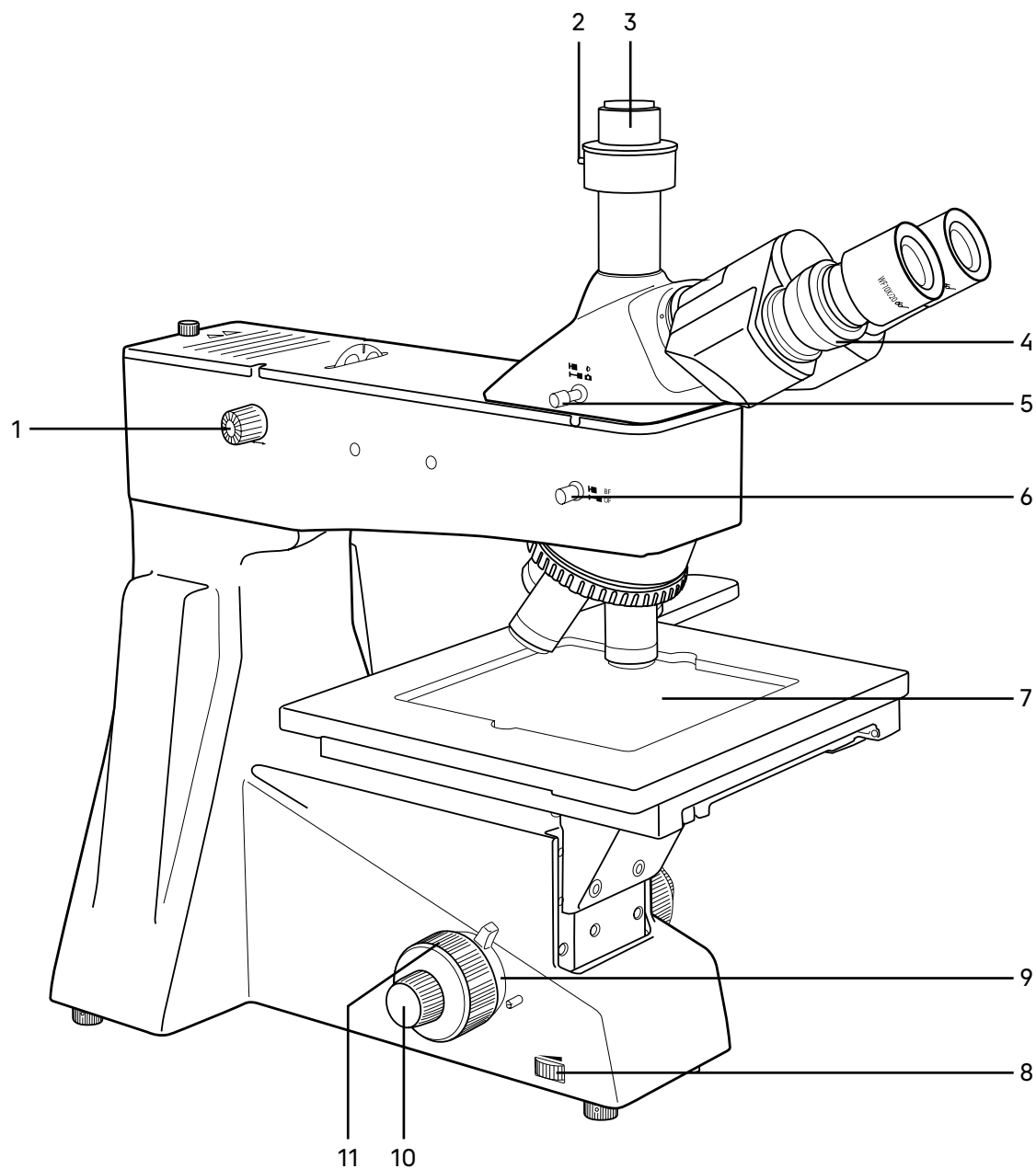
Рис. 2. Микроскоп MAGUS Metal D650 BD. Вид слева
