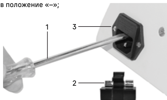
Рис. 19. Замена предохранителя
